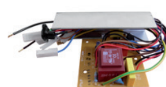
Platine für analoge BVC Zentralstaubsauger Artikel-Nr. 12352
